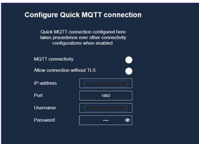
Abbildung 6: Benutzeroberfläche Gateway
