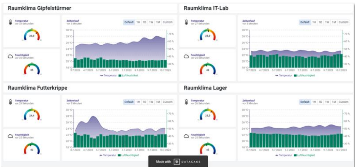
Abbildung 1: Dashboard Visualisierung
