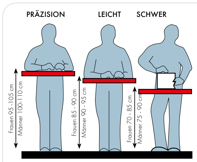
Stehendes Arbeiten
