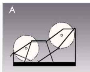
Bild A: Seitenansicht der Rollenständer. Ein Ständer kann 30 feste Boxen für 7"-Spulen mit einer Breite von 60 mm aufnehmen.
